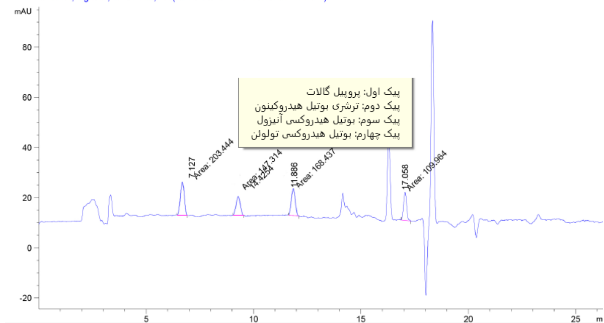
شکل-۱. کروماتوگرام ترکیبات آنتی‌اکسیدانی کل در ریزجلبک اسپیرولینا پلاتنسیس
