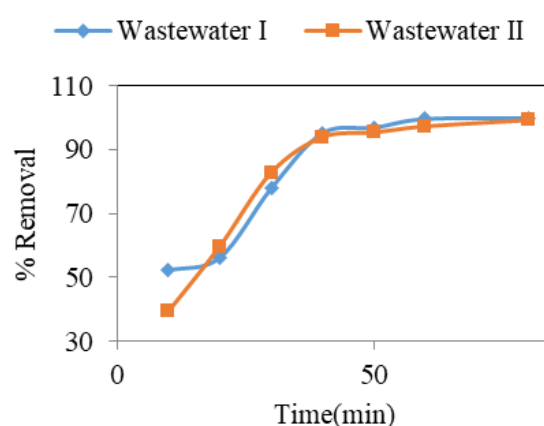
شکل-۸. تأثیر زمان تماس (۱۰، ۲۰، ۳۰، ۴۰، ۵۰، ۶۰ و ۸۰ دقیقه) بر ظرفیت جذب یون \text{NH}_4^+ (میلی گرم/گرم)
