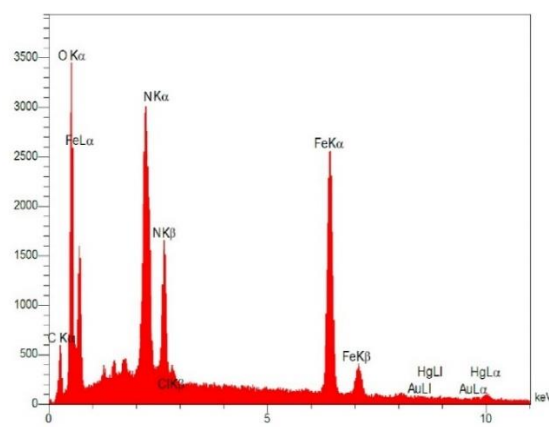
شکل ۵- آنالیز EDAX اثر جاذب هیدروژل نانو مغناطیسی پس از جذب پساب حاوی یون \text{NH}_4^+
