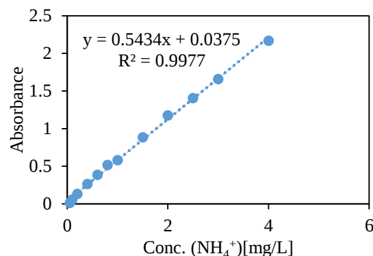
شکل ۱- نمودار کالیبراسیون جذب یون \text{NH}_4^+ دستگاه اسپکتروفتومتر UV در طول موج ۲۱۳ نانومتر
