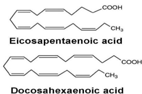
شکل-۱. ساختار اسیدهای چرب EPA (بالا) و DHA (پایین)
