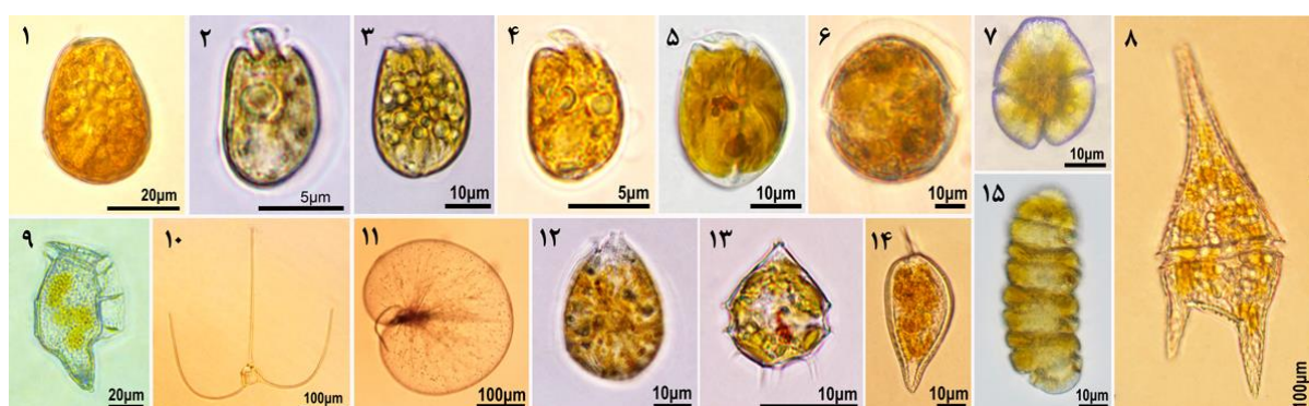
شکل - ۲. برخی از گونه‌های داینوفلاژله با پتانسیل تشکیل شکوفایی جلبکی مضر شناسایی شده در خلیج چابهار (دریای عمان) ۱: Prorocentrum lima , ۲: Amphidinium sp., ۳: A. operculatum , ۴: A. carterae , ۵: Amphidinium sp. 2, ۶: Scrippsiella trochoidea , ۷: Gyrodinium instriatum , ۸: Tripos furca , ۹: Dinophysis caudata , ۱۰: Tripos macroceros , ۱۱: Noctiluca scintillans , ۱۲: Ostreopsis sp., ۱۳: Peridinium quinquecorne , ۱۴: Prorocentrum micans , ۱۵: Cochlodinium polykrikoides (۹، ۱۰).
